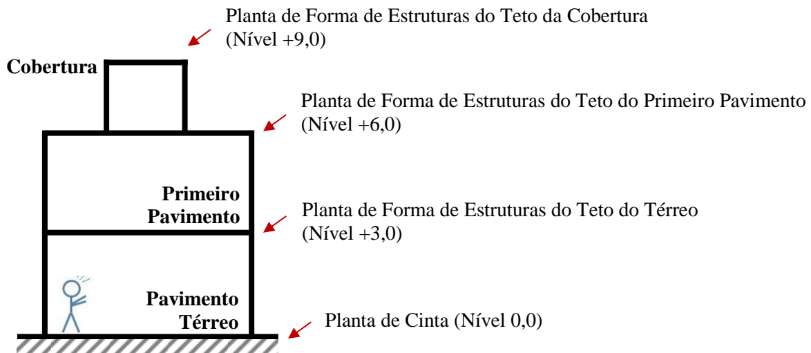
Corte do Edifício (Sem escala)
